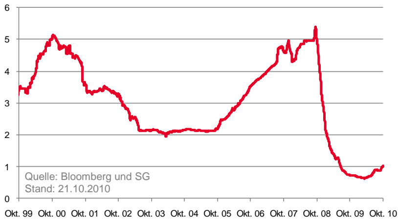
CHART 3-MONATS-EURIBOR 4
